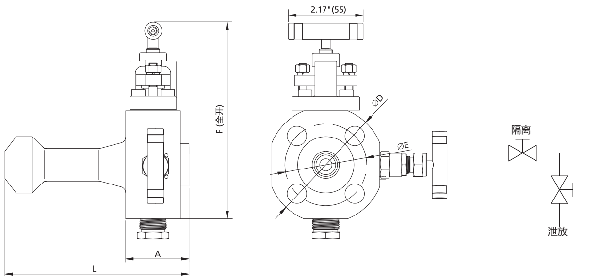
通径4mm阀体
