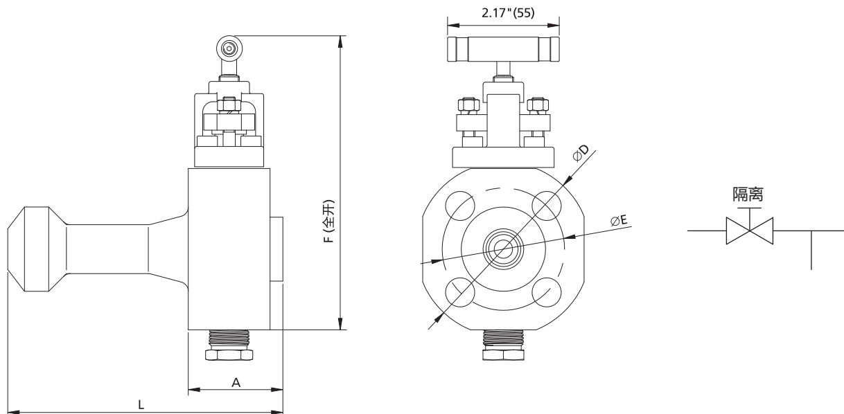
通径4mm阀体
