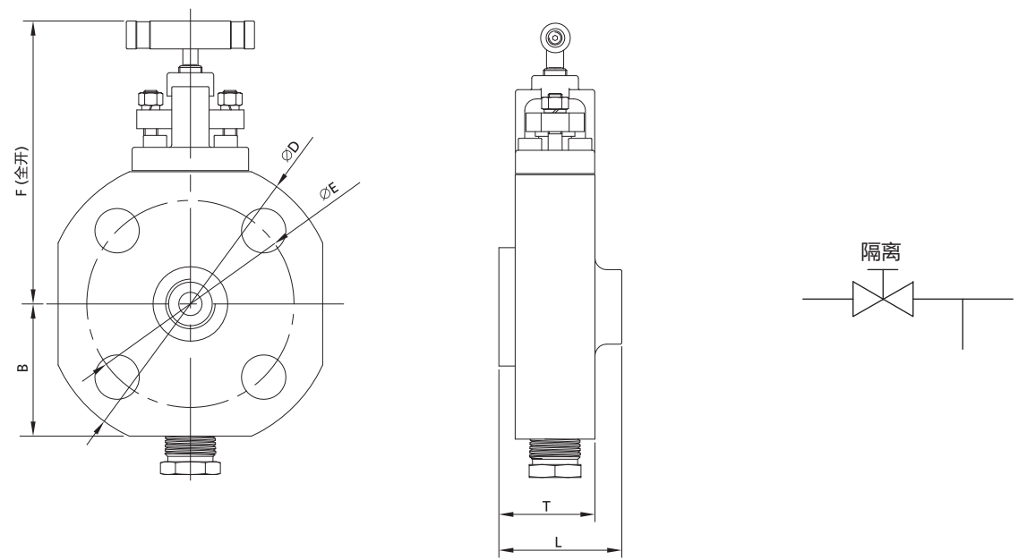
阀门组合形式 (O): OS&Y 针阀隔离, 带泄放口
