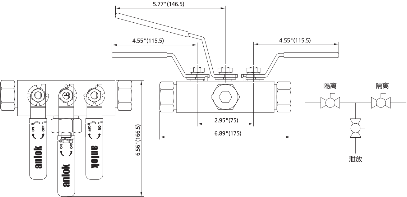
阀门组合形式 (BBB)：球阀隔离，球阀隔离，球阀泄放
