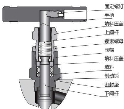
螺纹连接式阀帽针阀
