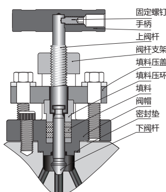
螺栓连接式明杆(OS&Y)针阀
