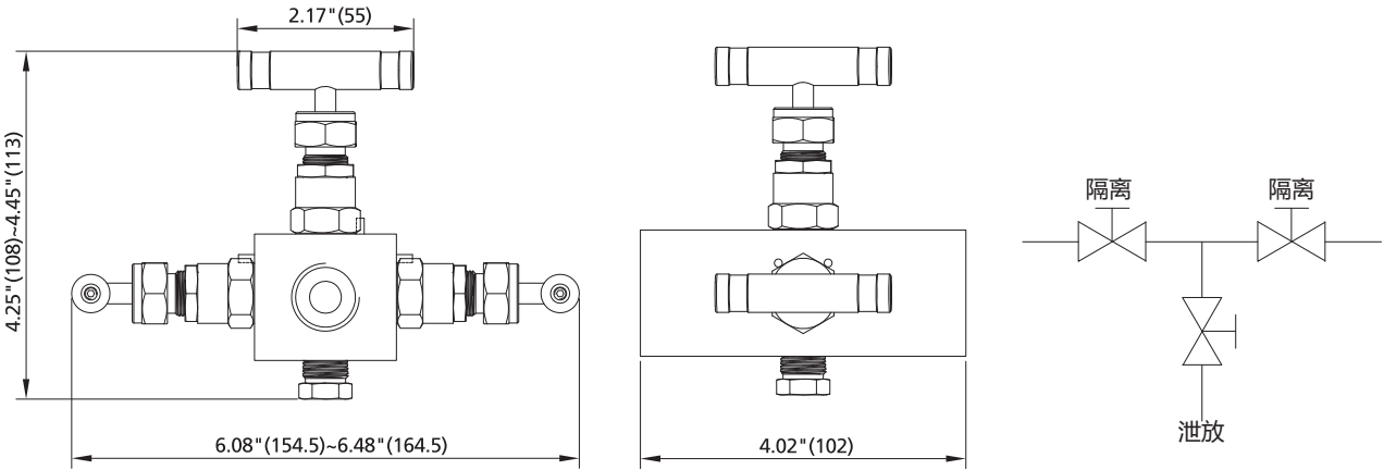
阀门组合形式 (NNN)：针阀隔离，针阀隔离，针阀泄放
