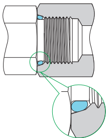
O型圈密封
