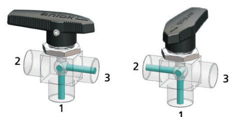
端口1,3连通
