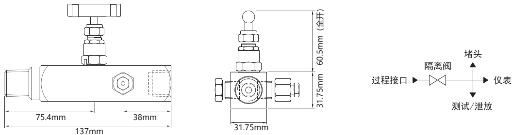
图示尺寸为GV1系列表阀的外形尺寸
