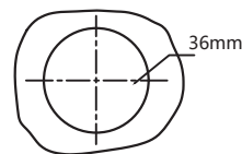
面板开孔尺寸
