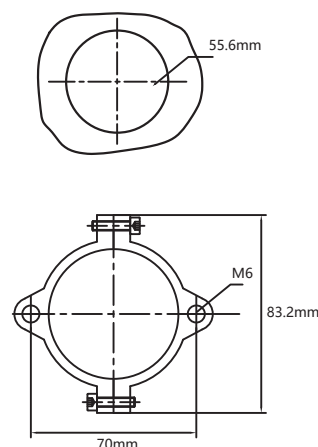
面板开孔尺寸
