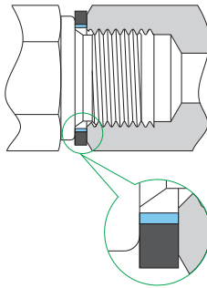
4.GA阳螺纹，根部复合垫片和FG阴螺纹
