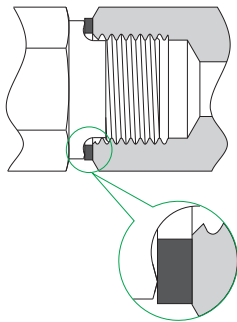
4.GA阳螺纹，根部复合垫片和FG阴螺纹
